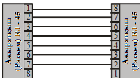
21- сурет. Консольдық кәбіл
