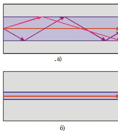
23 - сурет. Көпмодты(а) және бірмодты(б) талшық
